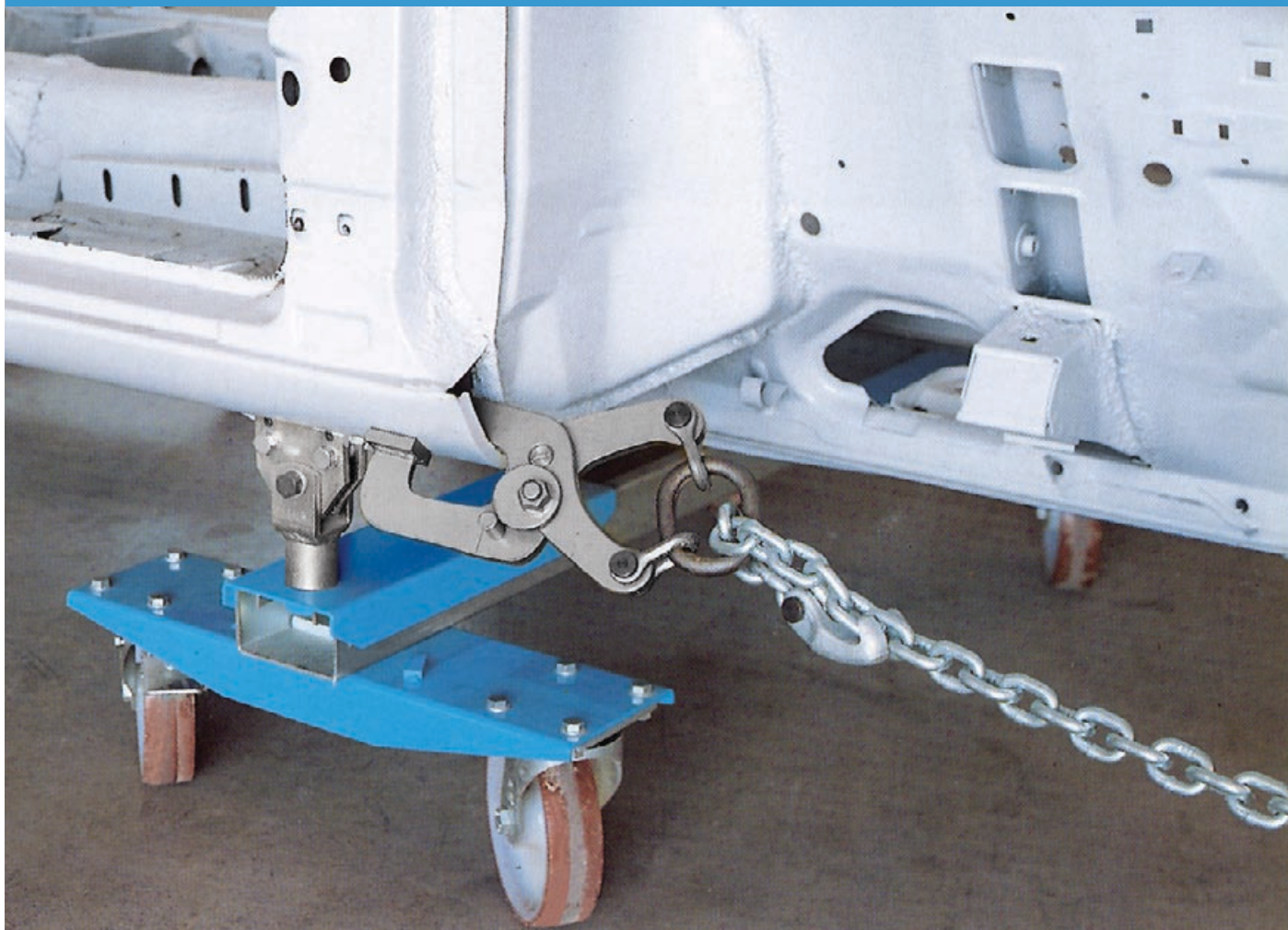
Art.144I Morsa.
